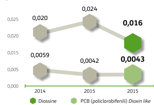
Figura 27 | Diossine e PCB (grammi tossicità equivalenti)
